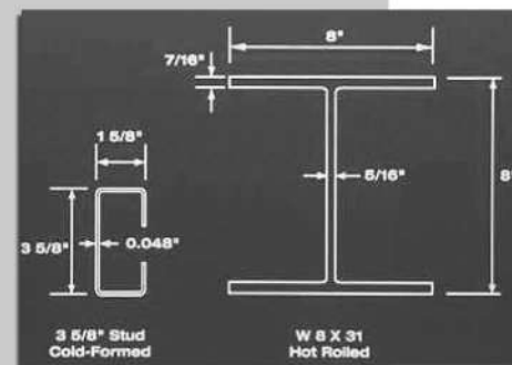
شکل ۸. فرم دادن ورق فلزی برای افزایش مقاومت
