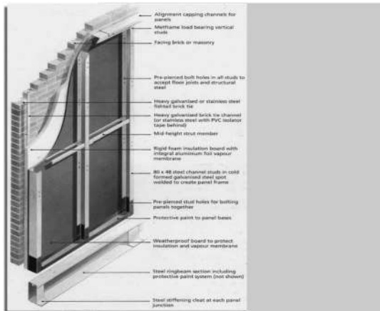
شکل ۱۰. شیوه ساخت دیوار در سیستم LSF
