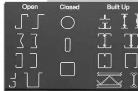
شکل ۹. CFS به نام‌های باز، بسته، ساخته‌شده
