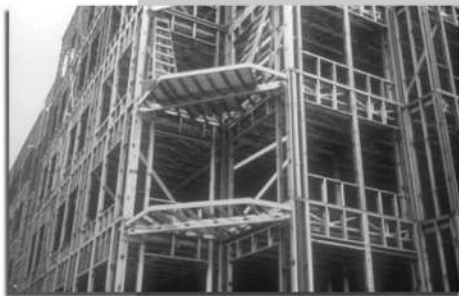
شکل ۱۱. سیستم LSF درجا
